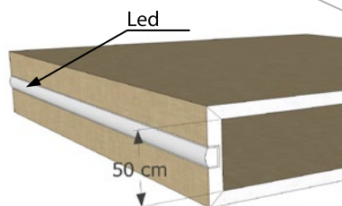
Art. M 05 Mensola o montante con inserimento del dissipatore in alluminio da voi richiesto
