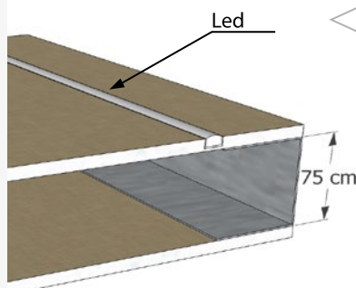
Art. M 06 Mensola o montante con inserimento del dissipatore in alluminio da voi richiesto
